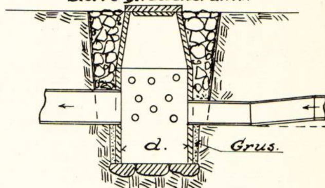
Större ylvattenbrunn.
