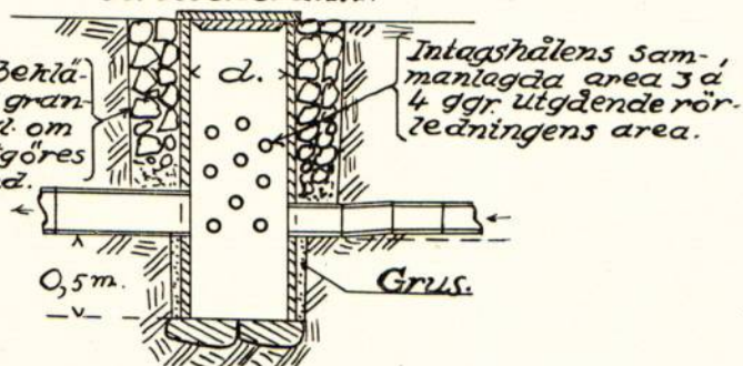
Ylvattenbrunn.
