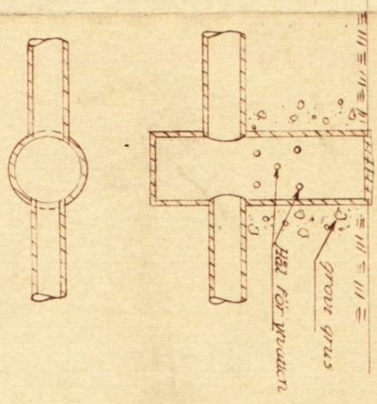
Förslag till brunn Skala 1:50
