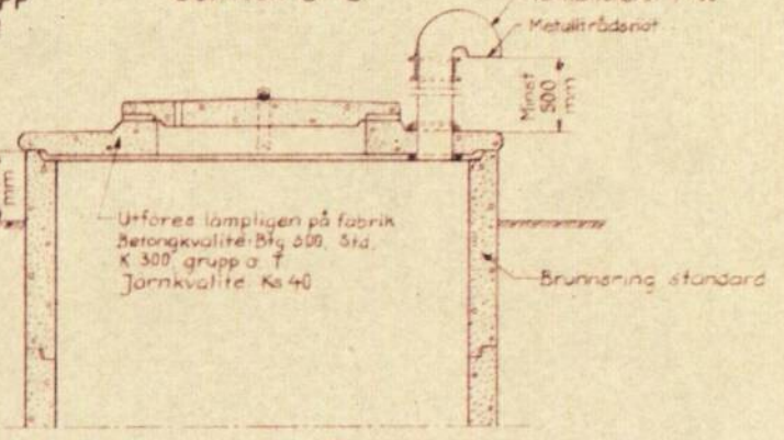
Sektion C - C
