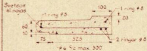
Plansektion A-A
