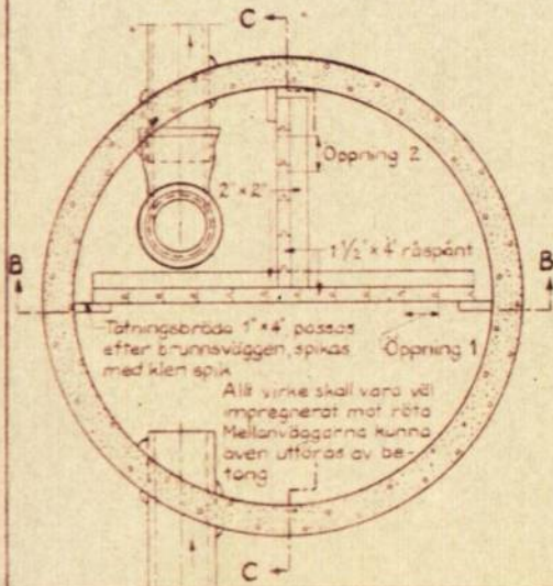
Plansektion A-A
