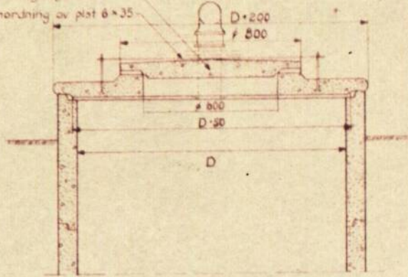
Sektion B - B
