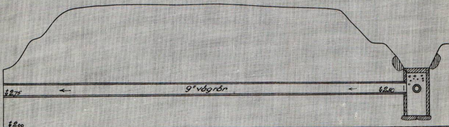
Genomlopp under landsväg vid I. Skala 1:50.
