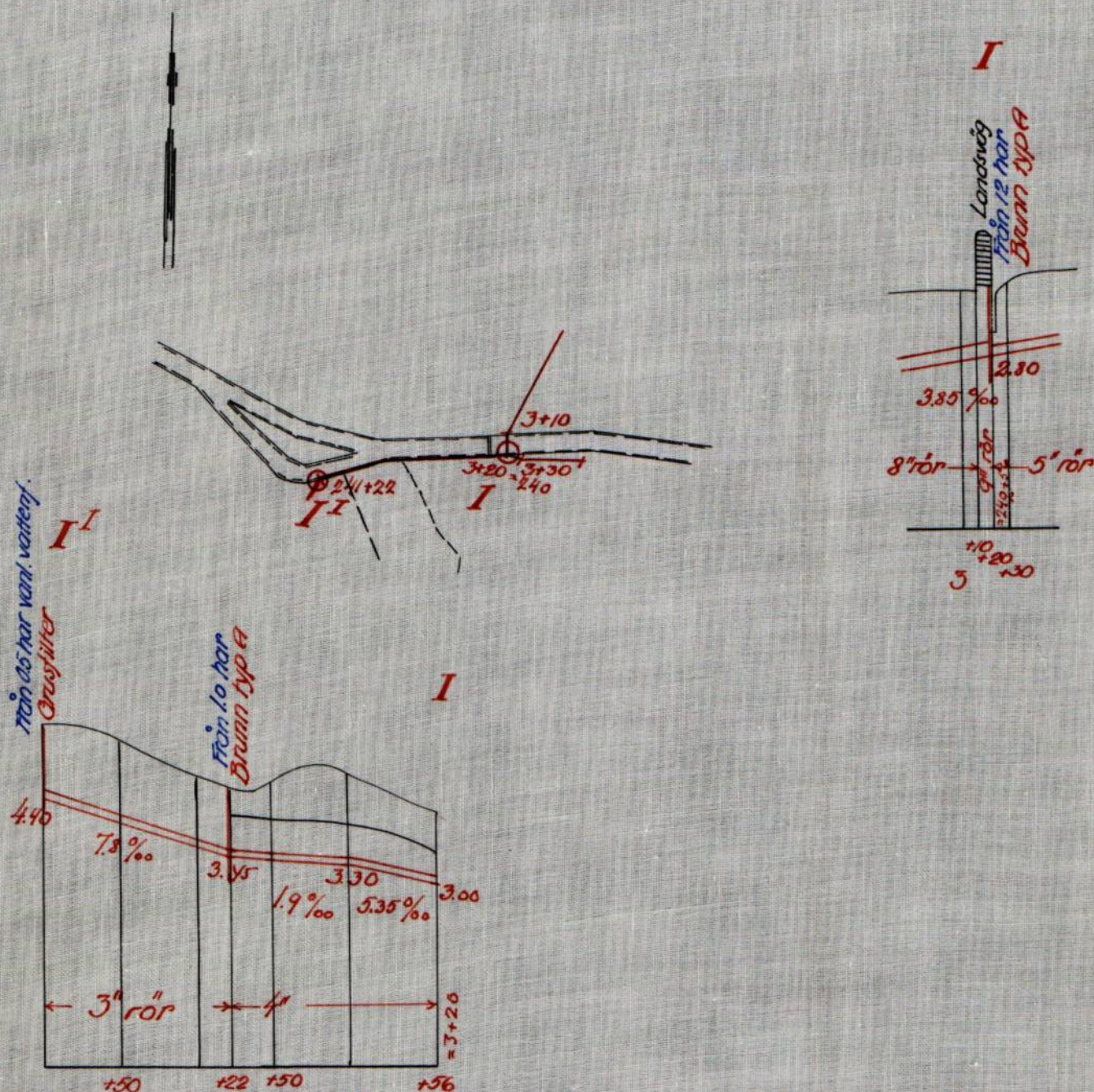
Genomlopp under landsväg vid I. Skala 1:50.
