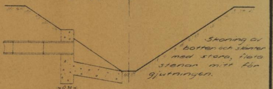
Betonggjutning typ B 2
