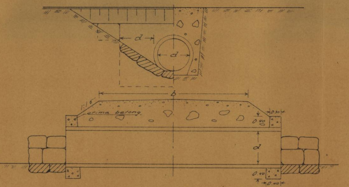
Rörtrumma typ A 2
