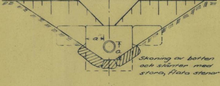
Betonggjutning typ A 2
