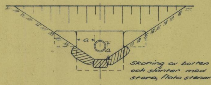
Betonggjutning typ A'
