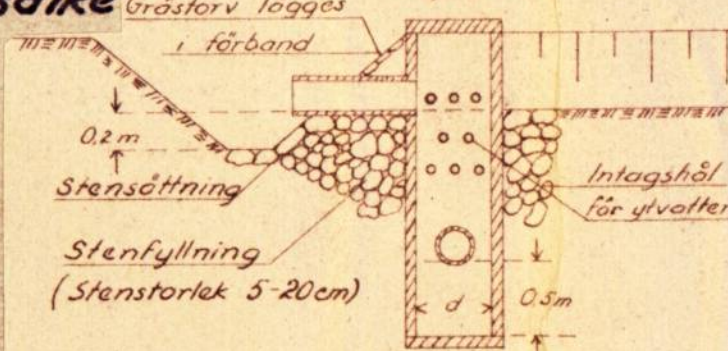
Betonggjutning vid rörutlopp under flödesdike
