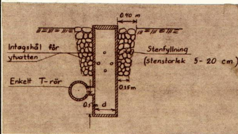
Brunn typ B-1 vid sidan av rörledning.
