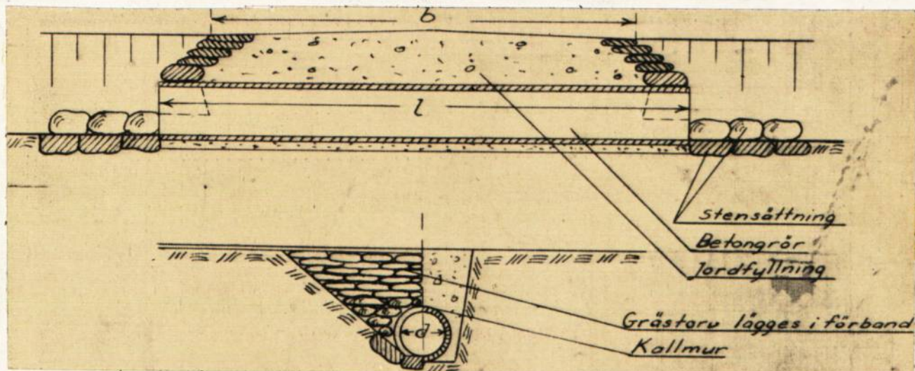
Trumma typ A.
