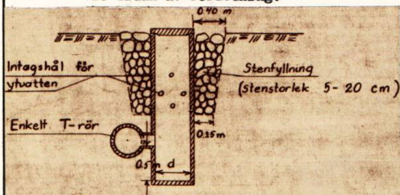
Brunn typ B-1 vid sidan av rörledning.
