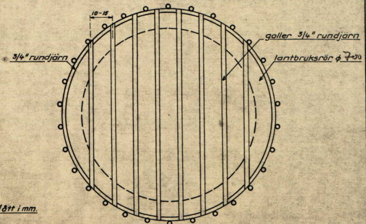
Sektion A-A.
