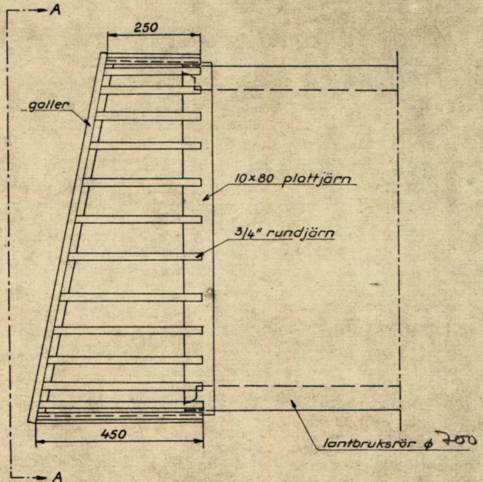
Sektion A-A.
