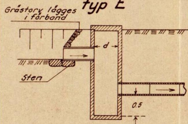
Betonggjutning vid rorutlopp under flödesdike
