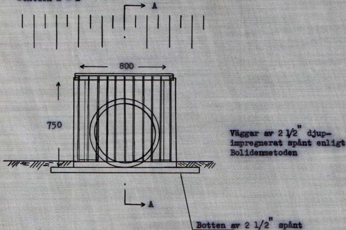
Sektion B - B
