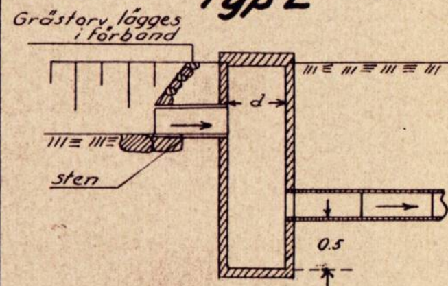
Betonggjutning vid rörtutlopp under flödesdike
