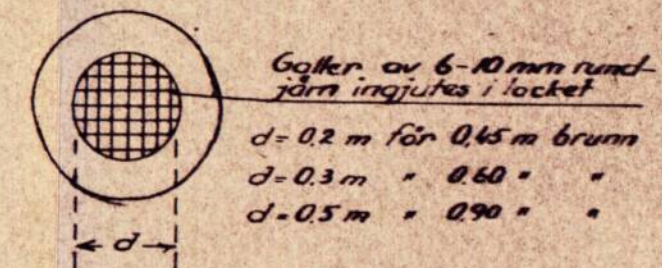
Detaljritning för lock med hål
