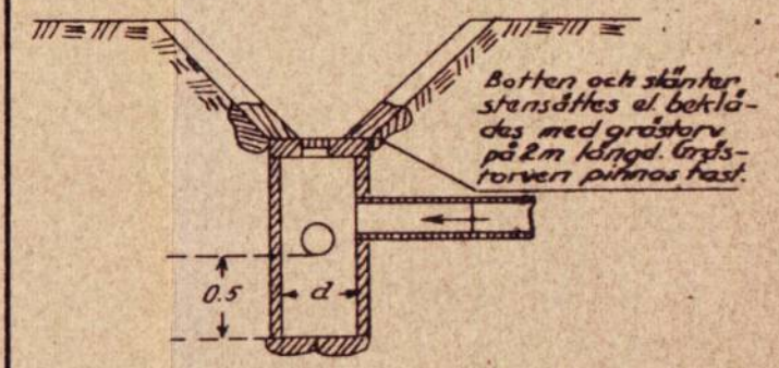
Detaljritning för lock med hål
