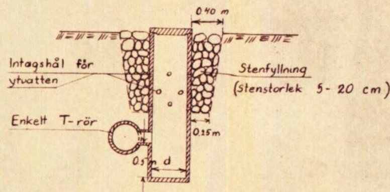
Brunn typ Ab vid sidan av rörledning
