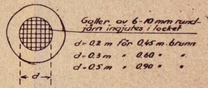
Detaljritning för lock med hål
