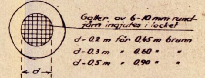
Detaljritning för lock med hål
