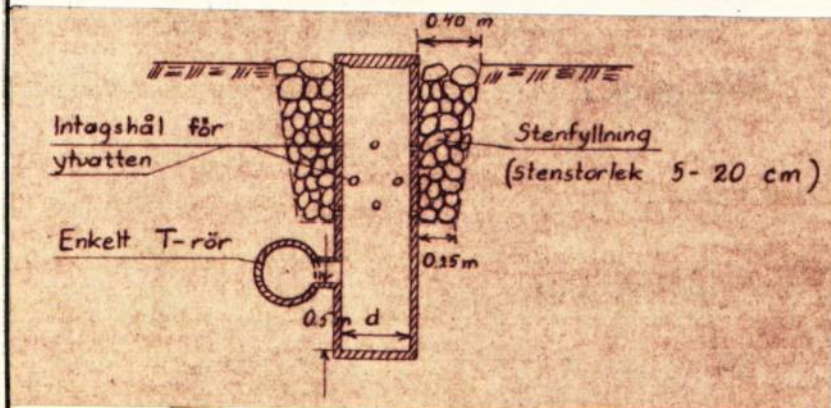
Brunn typ B-1 vid sidan av rörledning.
