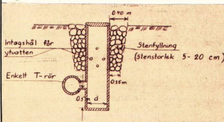
Brunn typ B-1 vid sidan av rörledning.
