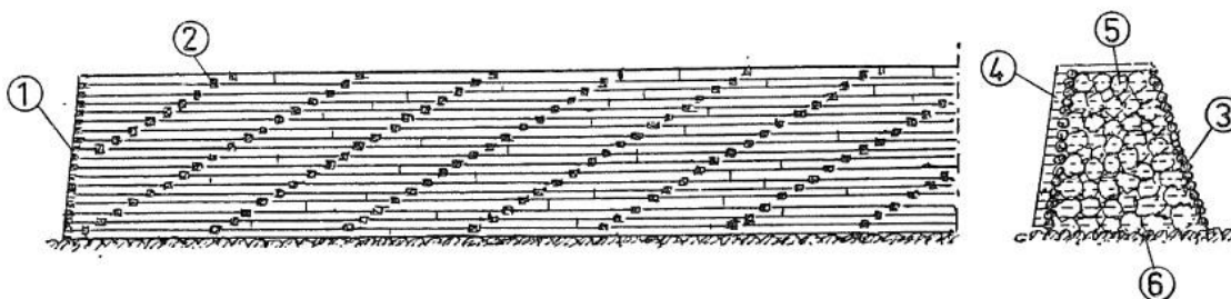
Figur 2: Skissen visar en dubbel träkistas uppbyggnad där bilden till vänster visar frontvåggen och bilden till höger visar kistan i genomskärning. 1: Uppströmsända, 2: Beting, 3: Frontvägg, 4: Bakvägg, 5: Stenfyllning och 6: Stenbotten. Källa: Skogsordlista 1969, Terminologicentrum TNC, Solna. Fd. Tekniska nomenklaturcentralen.
