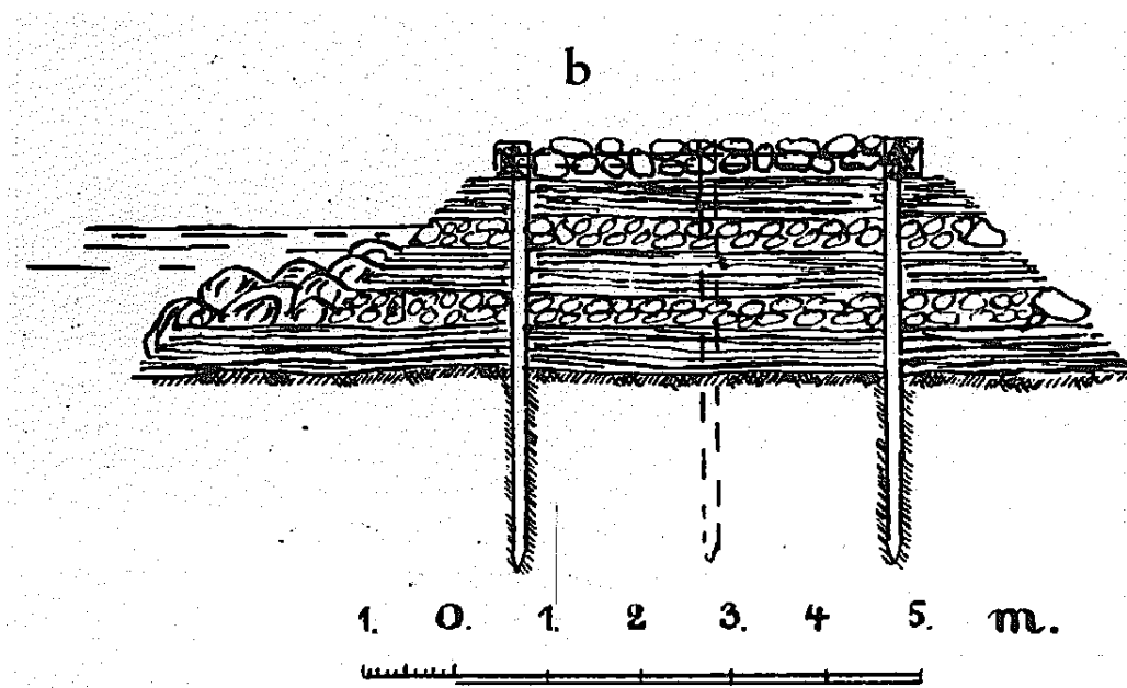
Figur 3. Teckningen visar en riskista i genomskärning. Denna är dessutom förstärkt med pålar. Källa: Norrlands Skogsvårdsförbunds Tidskrift 1917.
