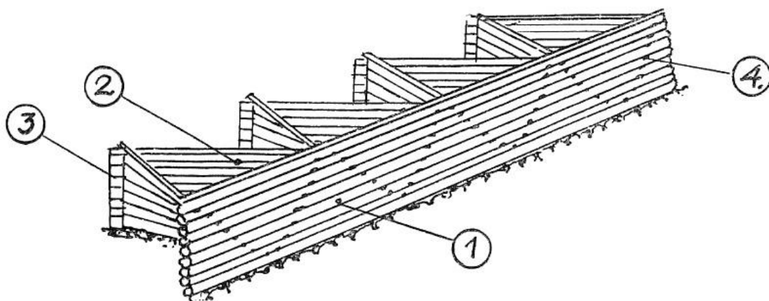
Figur 1: Illustrationen visar en enkel trækista där nr 1 är kistväggen, 2 trekantskaret, 3 en korsknut och 4 en laxknut. Källa: Skogsordlista 1969, Terminologicentrum TNC, Solna. F.d. Tekniska nomenklaturcentralen.
