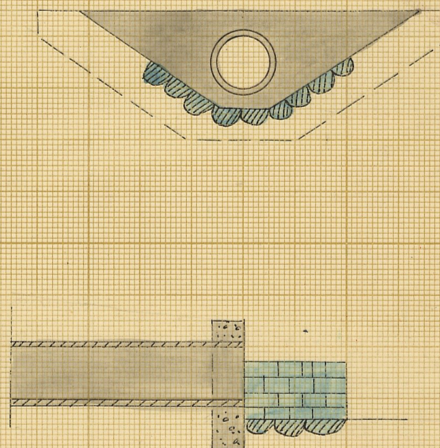
Dikesöga
