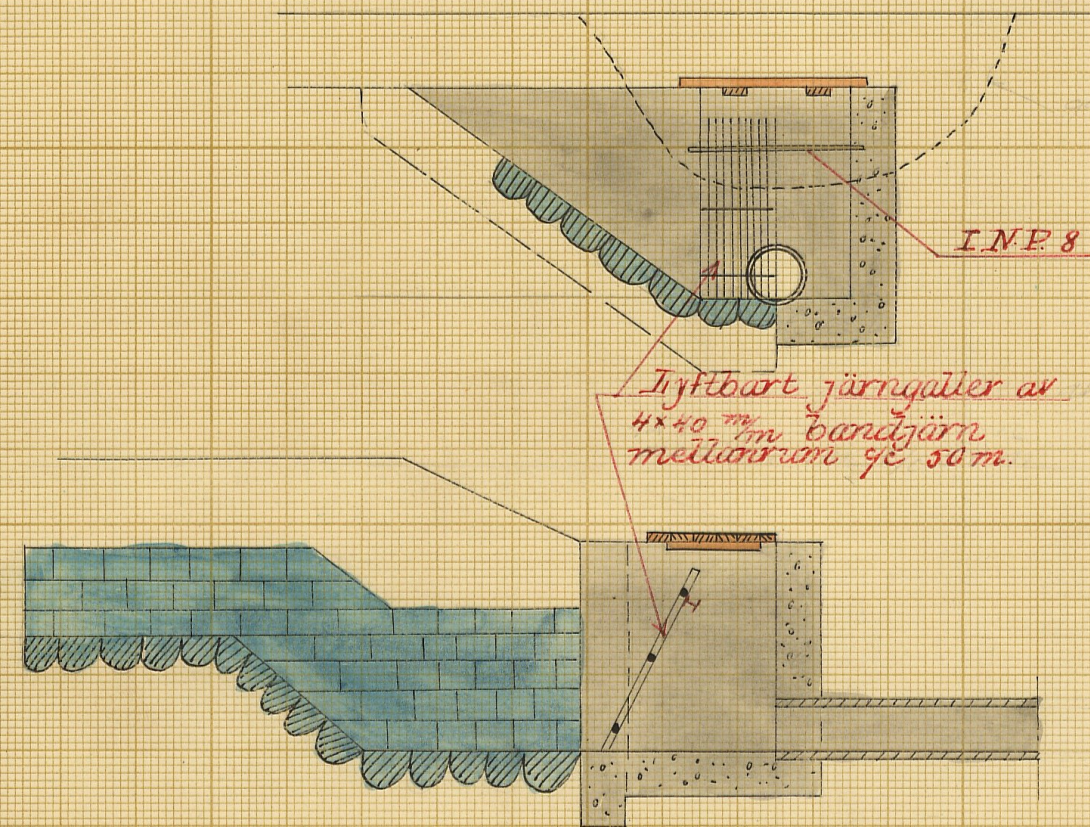
Intagningsbassäng
