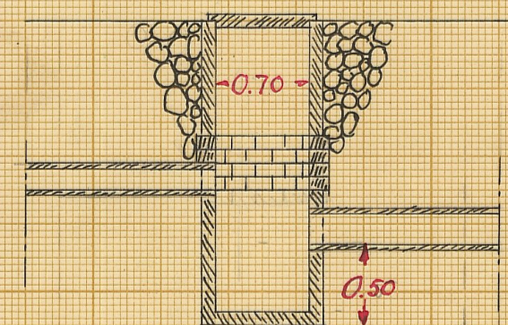
Förslag till intagningsbrunnar
