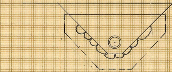
Förslag till dikesöga vid punkt 0 och 10+25
