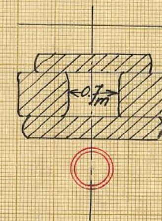
Sektion A-C
