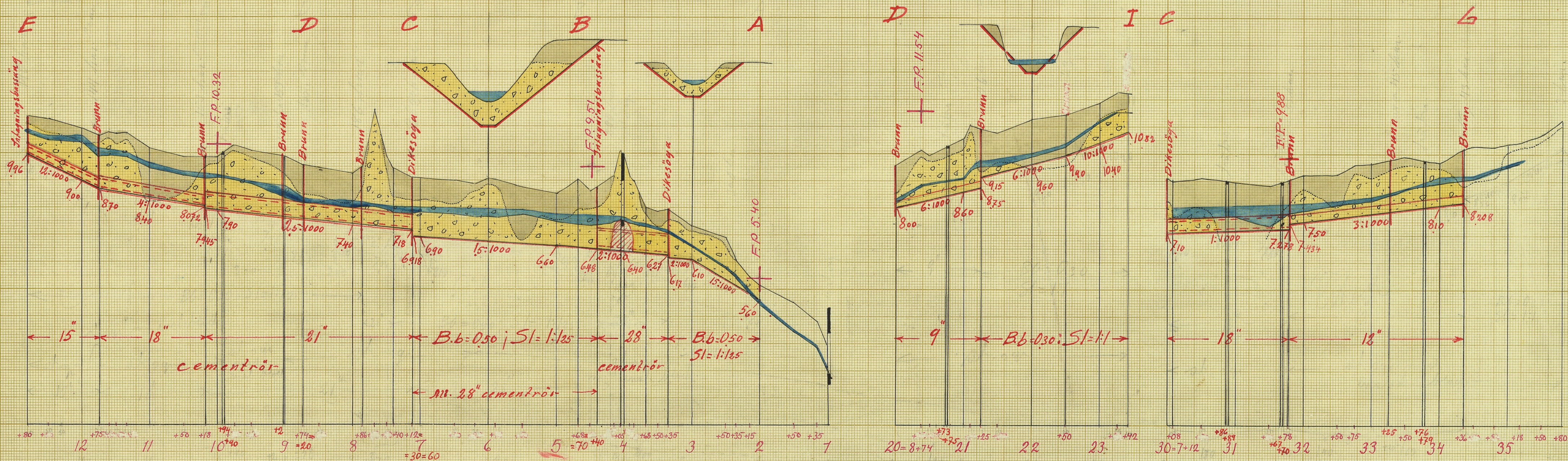
Längd-skala = 1:4000.
