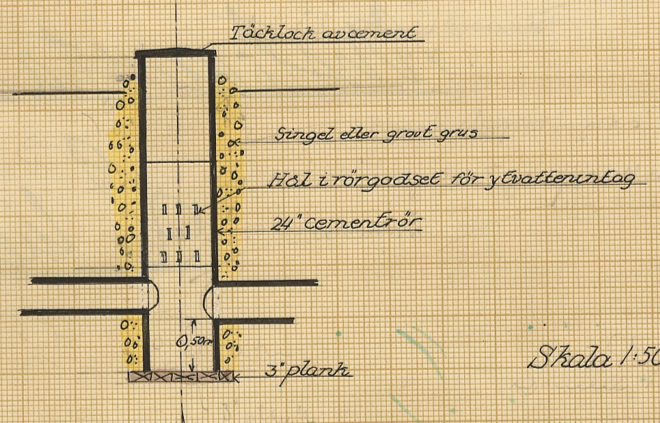
Typritning för intagsbrunn
