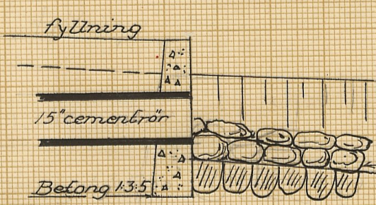
Rörutlopp vid sektion 1+30
