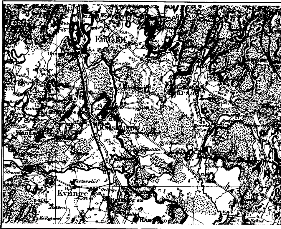
Kartblad nr 10 Karlshamn.
