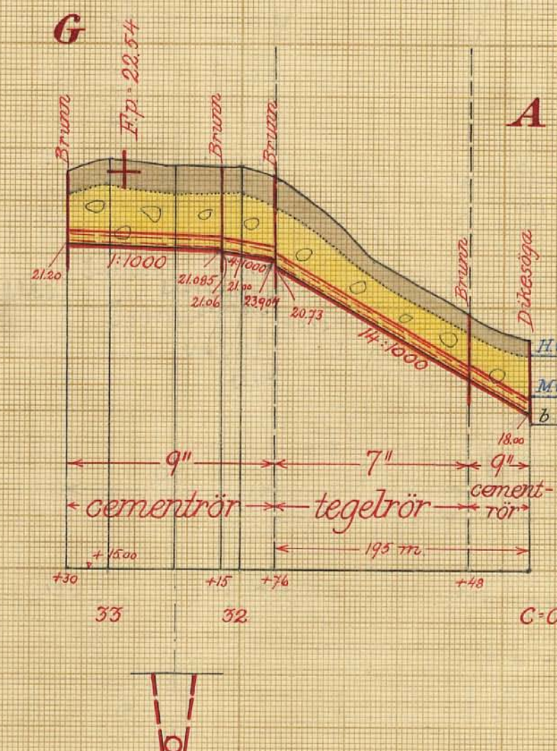
Typritning till dikesögon
