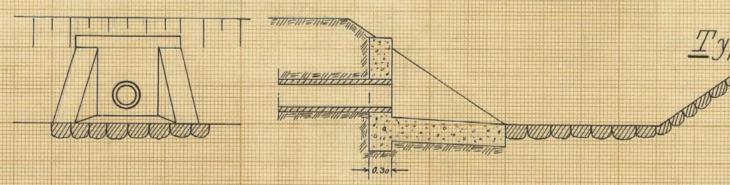
Typritning till dikesögon
