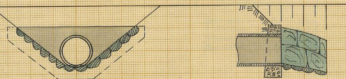
Förslag till dikesöga vid pkt 1+16
