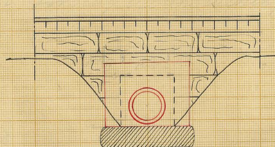
Allt. Förslag till anslutning vid järnvägstrumman
