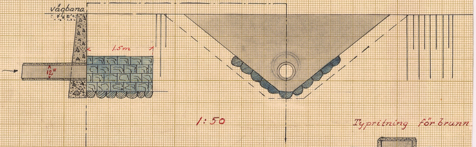
Förslag till dikesöga vid 0+62
