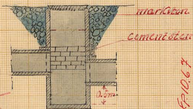
Förslag till Intagningsbrunnar
