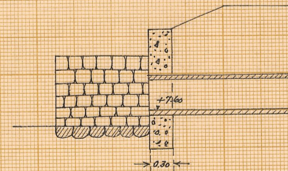
Typritning till dikesöga i punkt 0 +64
