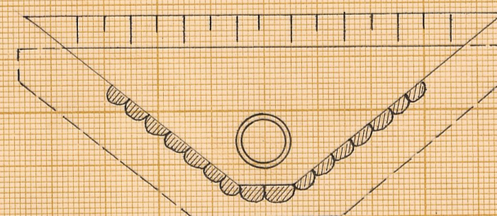
Typritning till dikesöga i punkt 0 +64
