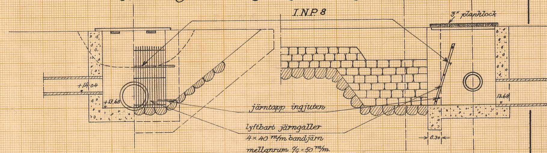
Typitning till intagningsbassäng i punkt 3 88
