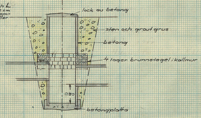
Typritning för brunn.
