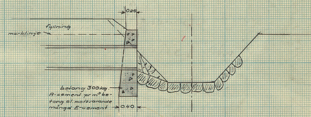
Rörlutlopp vid sekt. I+63.
