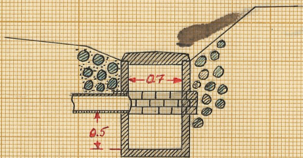
Förslag till intagningsbrunn.
