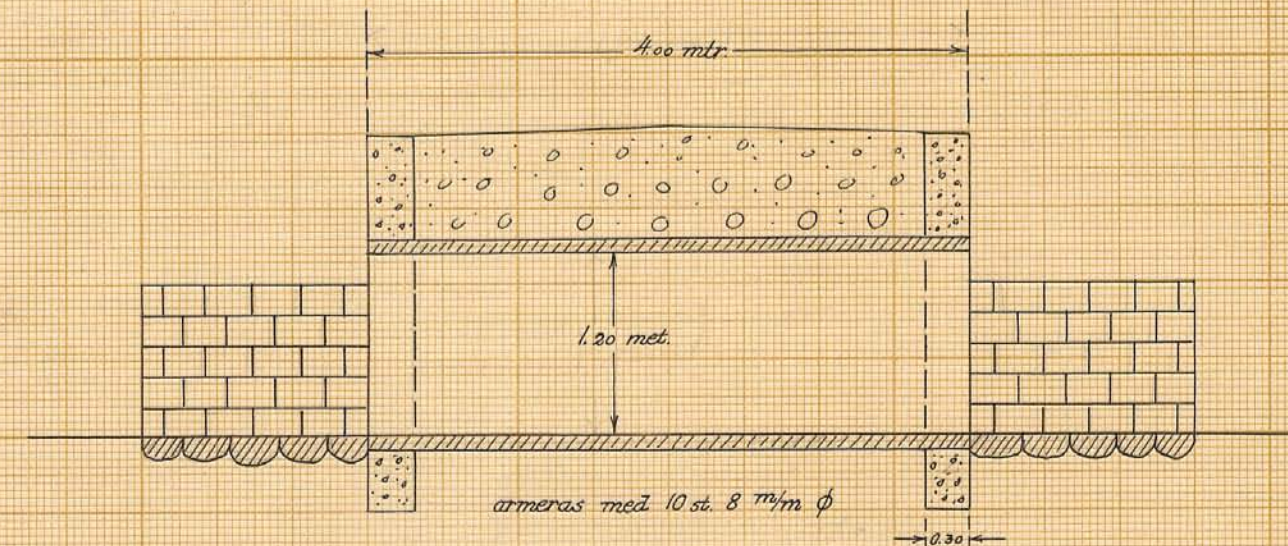
Typritning till betongkylvert vid 7+56, 8+40, 55+46 och 60+66
