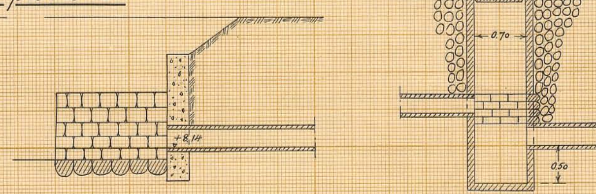
Typritning till intagningsbrunn
