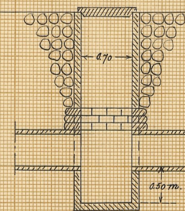
Typritning till intagningsbrunnar.
