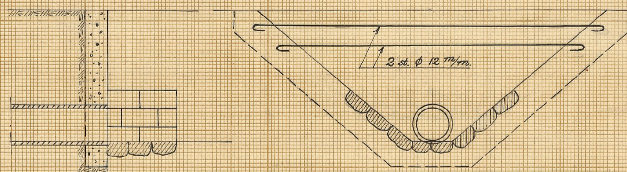
Förslag till dikesöga i punkt 0+35
