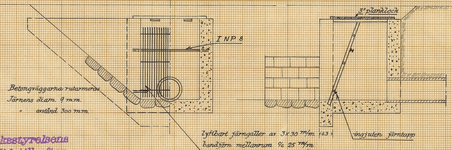
Förslag till intagningsbassäng i punkt 5+42
