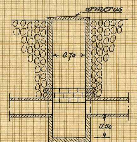
Typritning till intagningsbrunnar.
