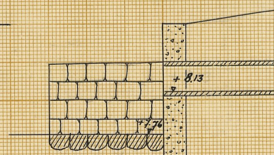
Förslag till dikesöga vid punkt 1 +20 .
