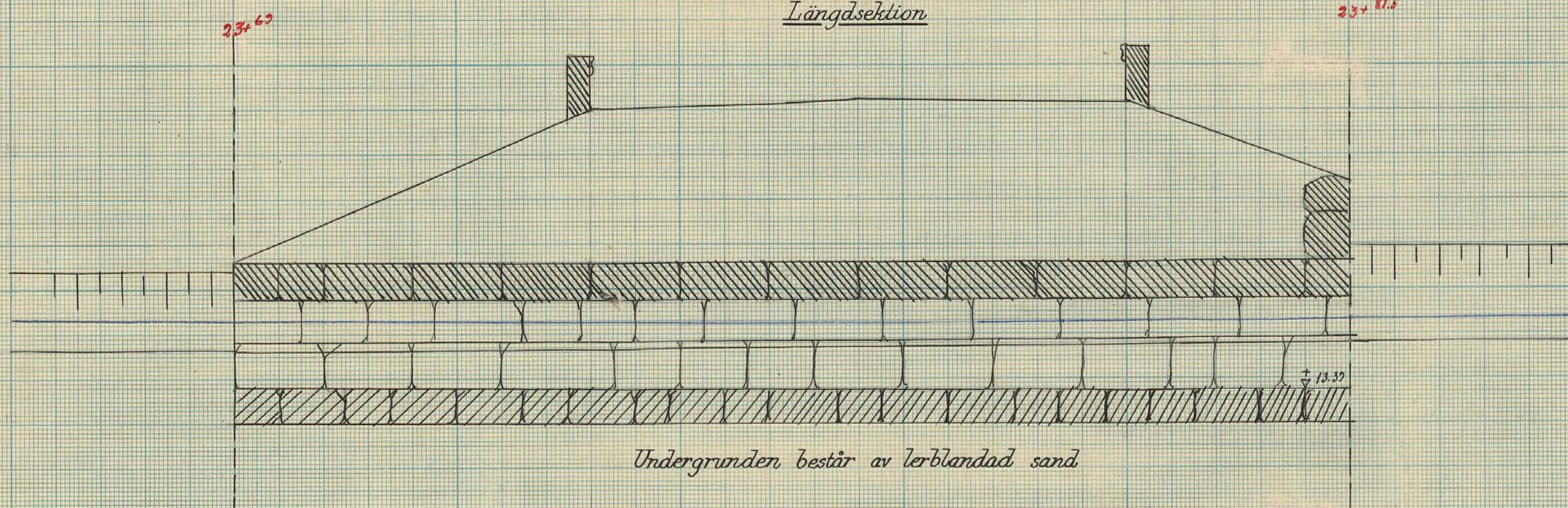
Längdsektion
