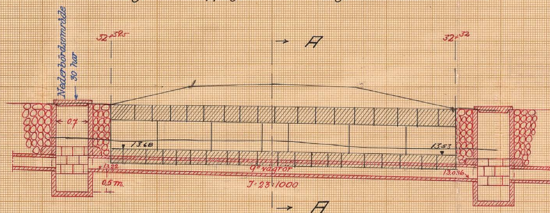
Förslag till avlopp genom landsvägen vid 32+32-32+39.5
