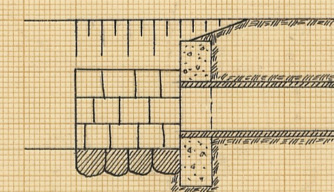
Betongmuren rubarmeras. Järnens diameter = 8 mm avstånd = 250 mm
