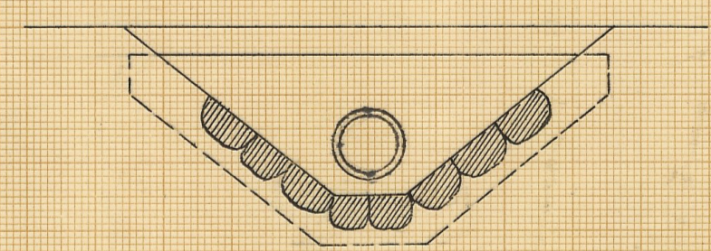
Förslag till dikesöga vid 6+63
