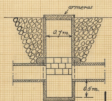
Typritning till intagningsbrunnar vid 7+02.12+54
