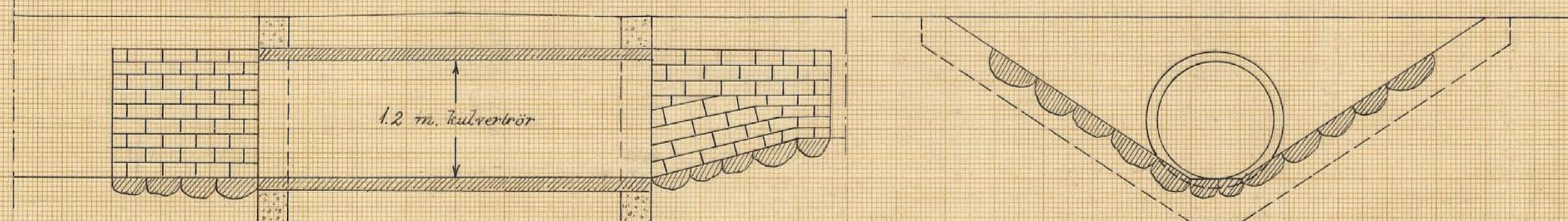
Förslag till brokulvert vid 8 +38 -8 +42 .
