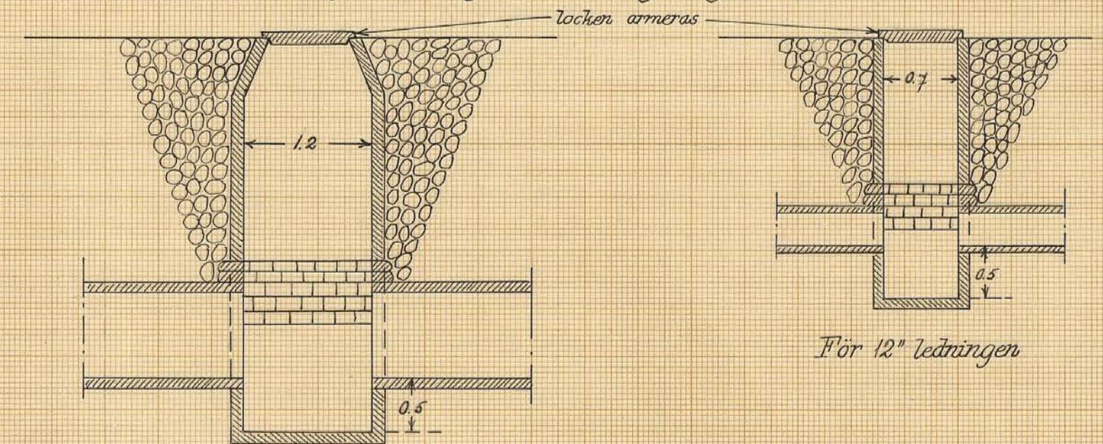
För 32" ledningen
