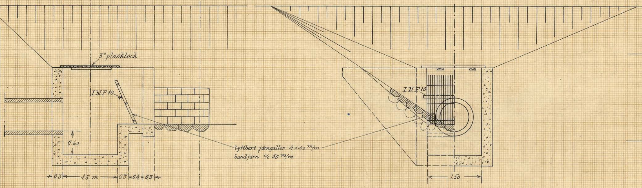
Förslag till intagningsbassäng vid 2 +70 .
