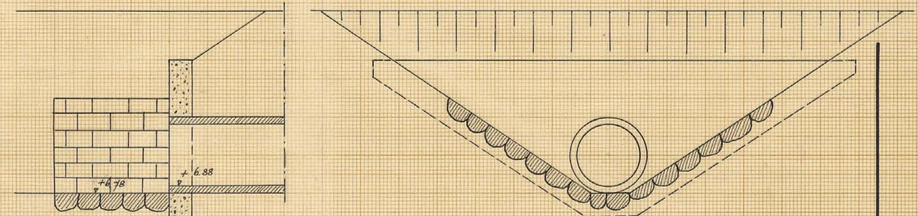
Förslag till dikesöga vid 0 +40 .
