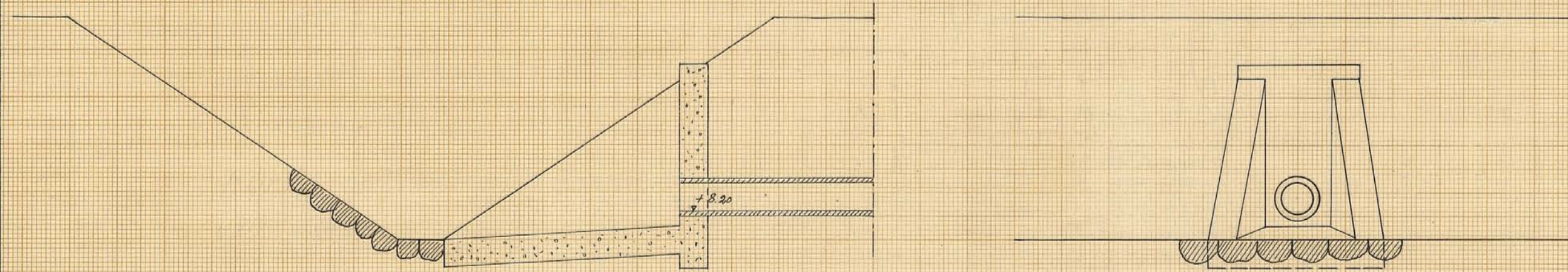
Förslag till dikesöga vid 10 +00 .
