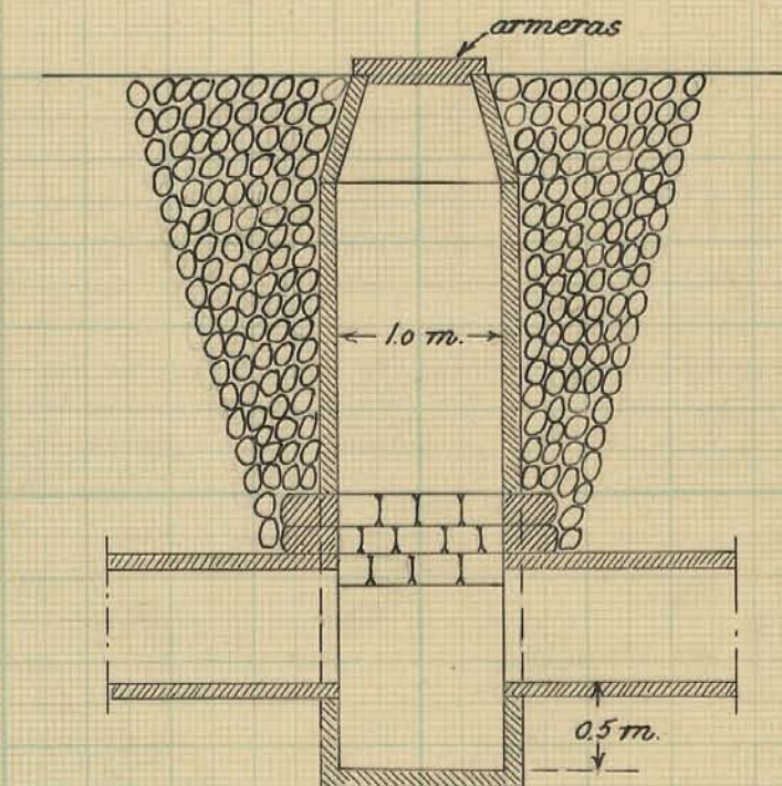
Förslag till intagningsbrunn vid 2+16
