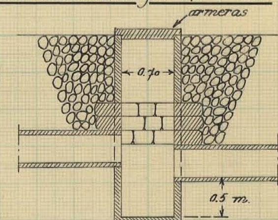
Typritning till intagningsbrunnar vid rörledningar \phi 9"-18"
