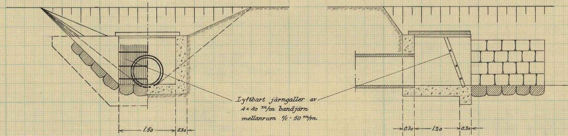
Förslag till dikesöga vid 6+15
