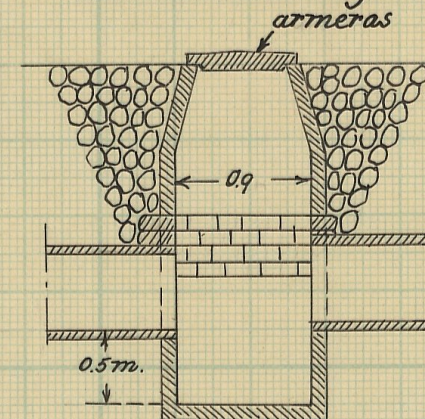
Typritning till intagningsbrunnar för 21" ledningen
