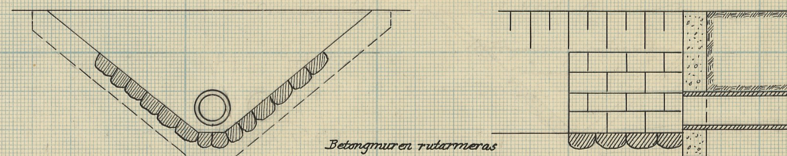
Förslag till dikesöga vid 1+00.
