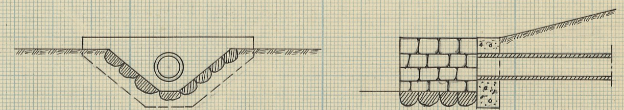
Förslag till rörutlopp vid A.
