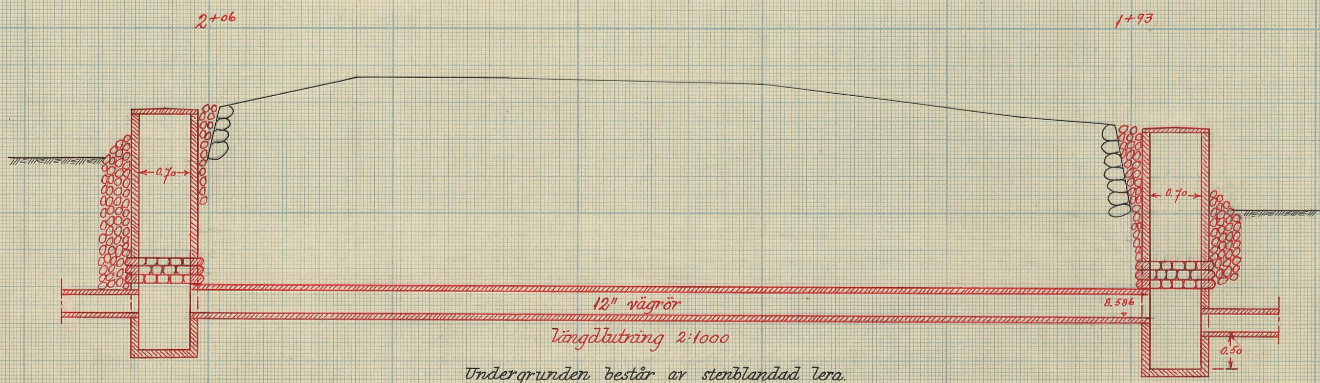
Förslag till rörledning genom allmänna vägen Bjärlöv - Torsebro.
