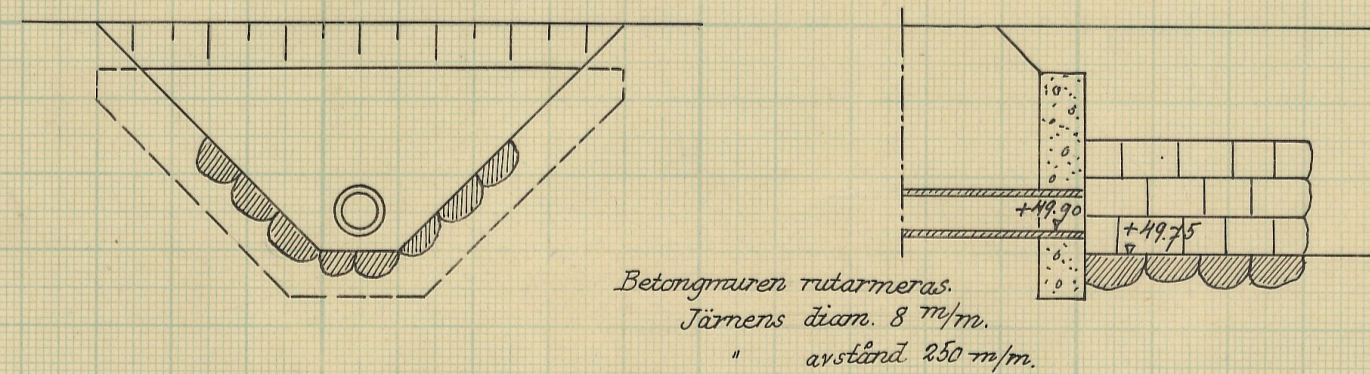
Typritning till intagningsbrunnar.
