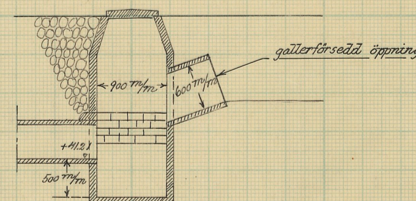
Förslag till intagningsbrunn vid 1+97.
