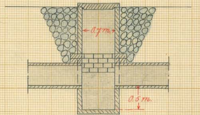
Förslag till intagningsbrunn
