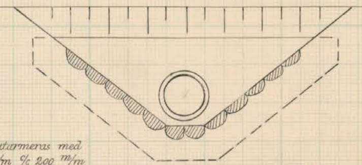
Förslag till dikesöga vid 1+45
