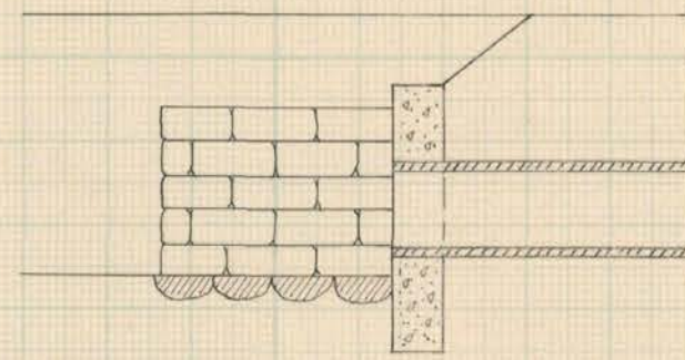
Förslag till dikesöga vid 1+45
