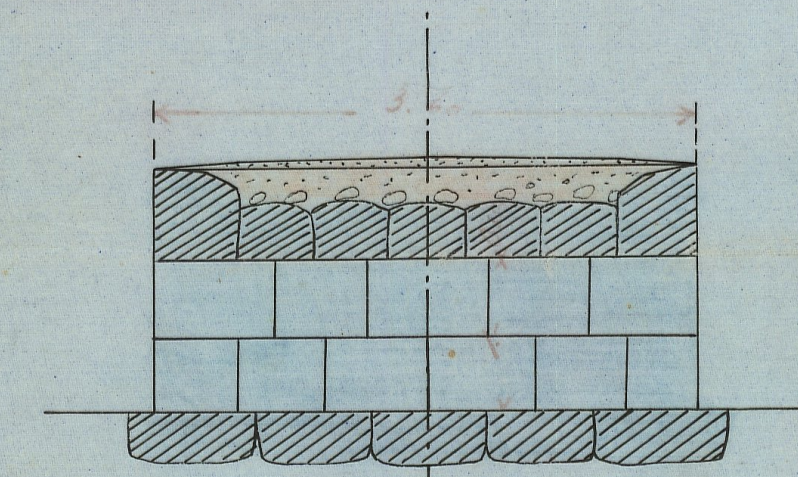
Förslag till väst-vägg.
