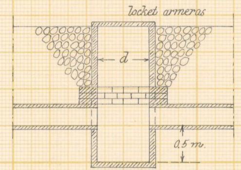
Typritning till intagningsbrunn
