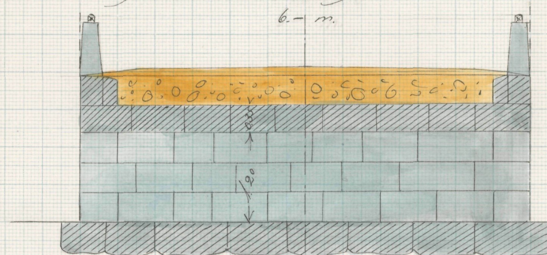
Förelag till landvägstrumman vid 4+75
