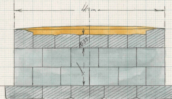
Förelag till ägervägsturmma vid 1+50
