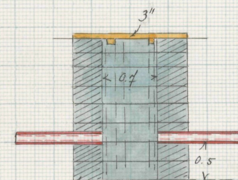
Förelag till intagningsbrunn
