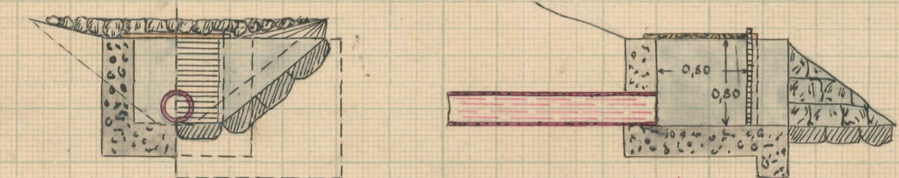
Förslag till dikesöga vid p. lock 2+25
