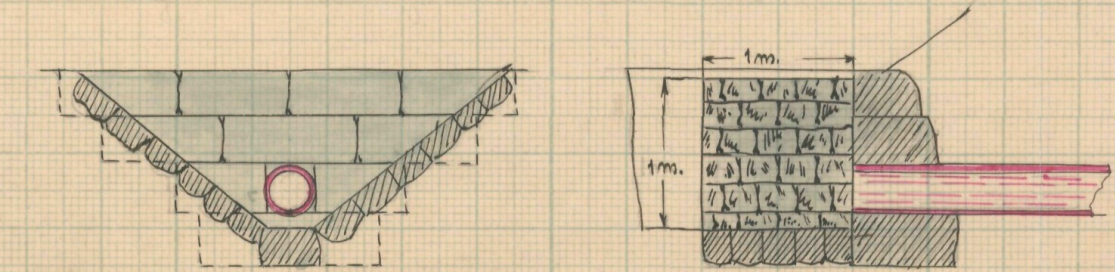
Förslag till dikesöga vid punkt 5
