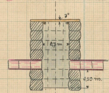
Förslag till dikesöga vid p. lock 2+25
