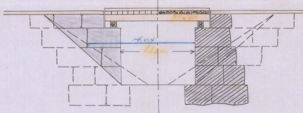
Förslag till utbyggnad vid 24+51
